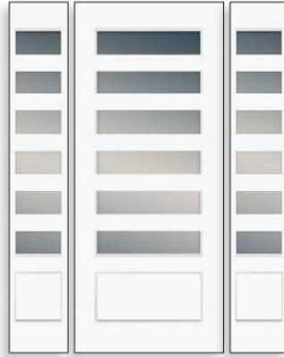
Door: 3/0 6/8 2648-010-C-1-SO3-6H Sidelites: 1/2 6/8 848-010-C-1-SO3-6H
