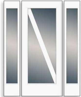
Door: 3/0 6/8 2664-010-C-X-SO4-22DIAB Sidelites: 1/2 6/8 764-010-C-X
