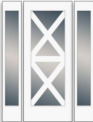
Door: 3/0 8/0 2680-010-C-X-SO3-2XBUK Sidelites: 1/2 8/0 880-010-C-X
